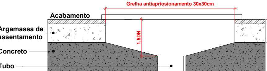
CORTE
