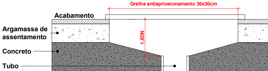
CORTE
