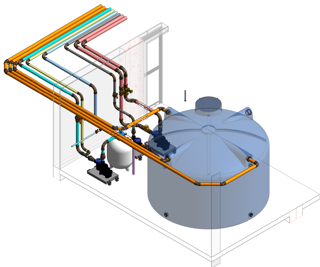
CASA DE BOMBAS - FRIENDS & POOL 1:50
