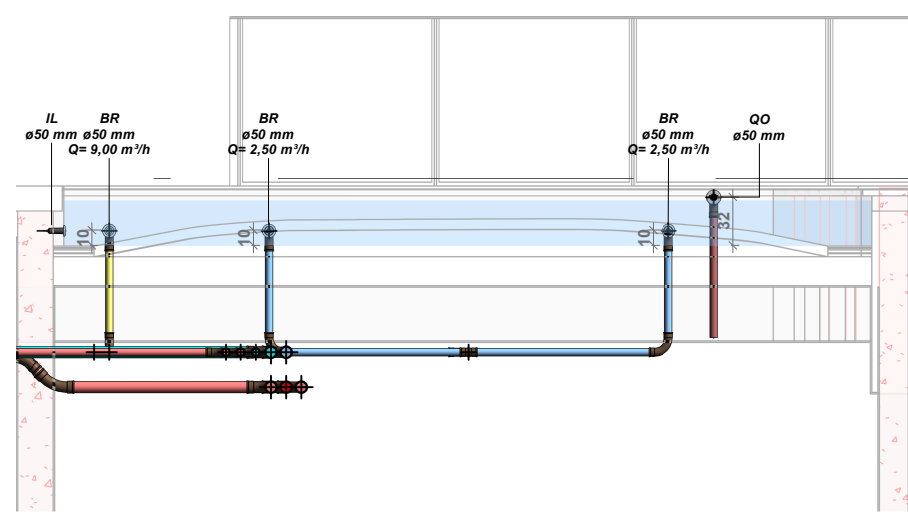
CORTE BB - SPLASH KIDS 1:50
