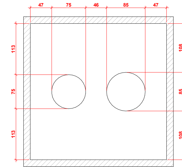
PLANTA BAIXA
