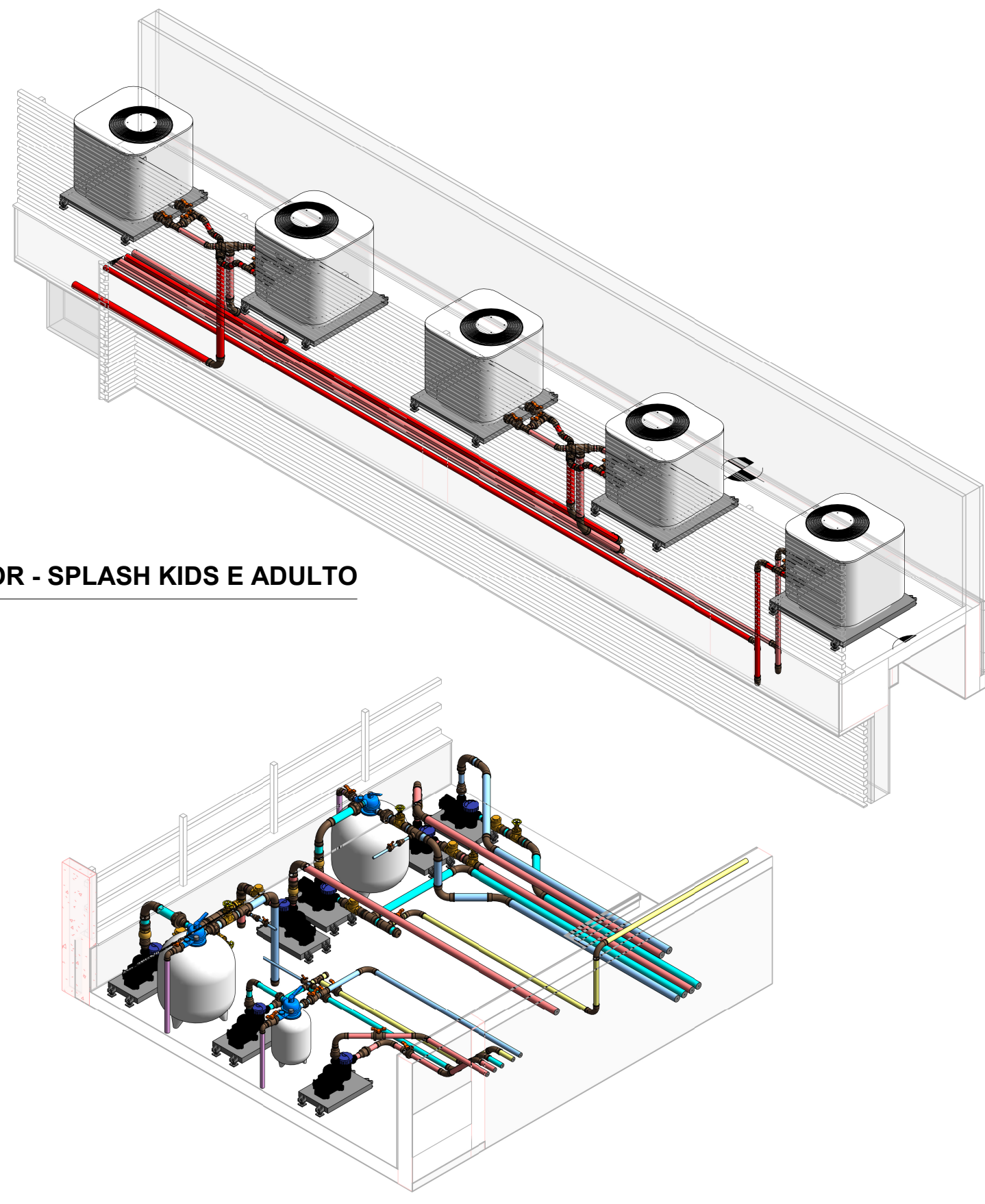
CASA DE BOMBAS - SPLASH KIDS E ADULTO 1:50
