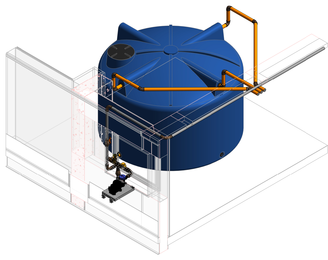
ÁREA TÉCNICA RESERVATÓRIO BORDA INFINITA - PISCINA ADULTO 1:50
