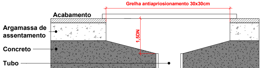
CORTE
