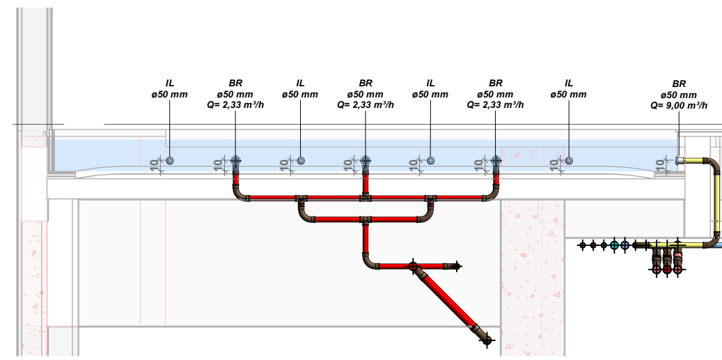
CORTE CC - SPLASH KIDS 1:50
